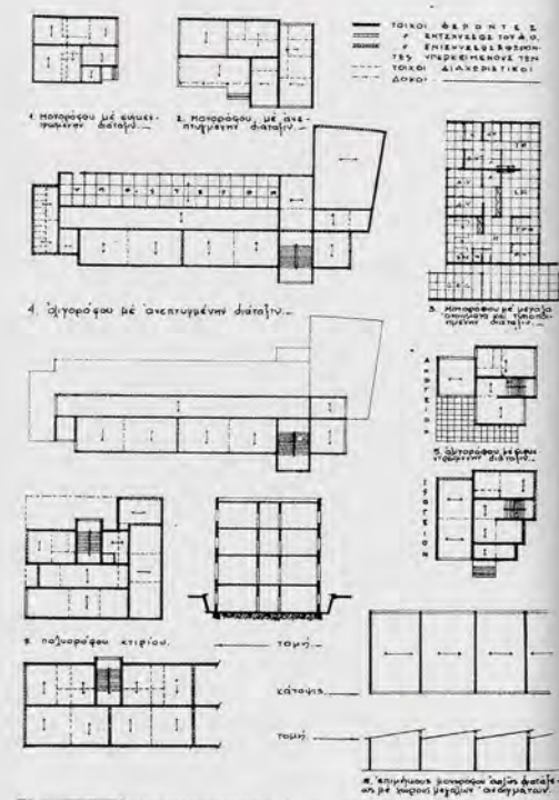
ΠΙΝΑΞ 3. — ΓΕΝΙΚΑΙ ΔΙΑΤΑΞΕΙΣ ΦΕΡΟΝΤΩΝ ΟΡΓΑΝΙΣΜΩΝ ΚΤΙΡΙΩΝ ΜΕ ΣΤΟΙΧΙΑ ΚΑΤΑΚΟΡΥΦΑ ΕΚ ΤΟΙΧΩΝ
