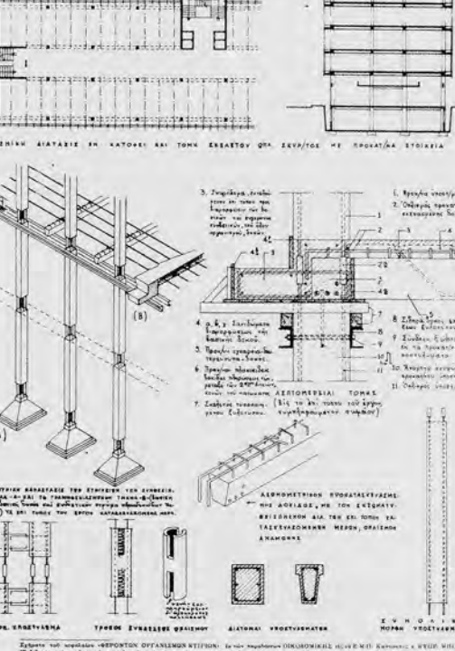
ΠΙΝΑΞ 24. — ΔΙΑΜΟΡΦΩΣΙΣ ΚΑΙ ΛΕΠΤΟΜΕΡΕΙΑΙ ΣΥΓΚΡΟΤΗΣΕΩΣ ΚΑΙ ΚΑΤΑΣΚΕΥΗΣ ΚΤΙΡΙΩΝ ΕΚ ΤΥΠΟΠΟΙΗΜΕΝΩΝ ΚΑΙ ΠΡΟΚΑΤΑΣΚΕΥΑΣΜΕΝΩΝ ΣΤΟΙΧΕΙΩΝ ΟΠΛΙΣΜΕΝΟΥ ΣΚΥΡΟΔΕΜΑΤΟΣ
