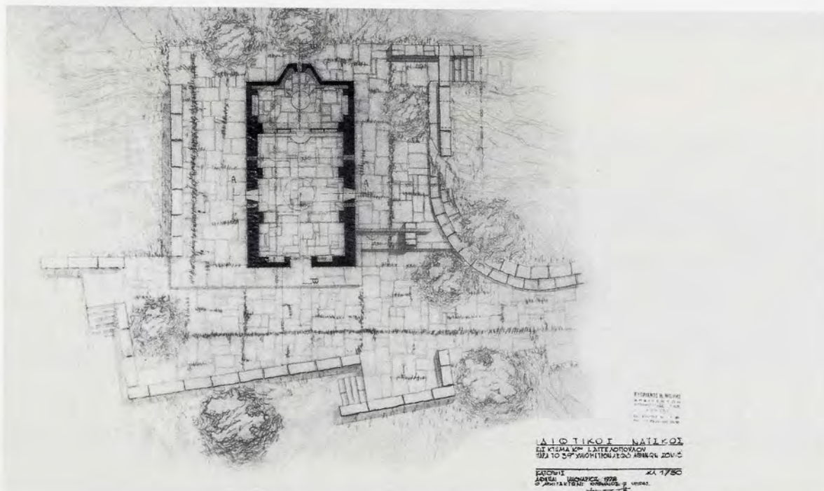
Κάτοψη ναΐσκου Σχέδια με μολύβι
