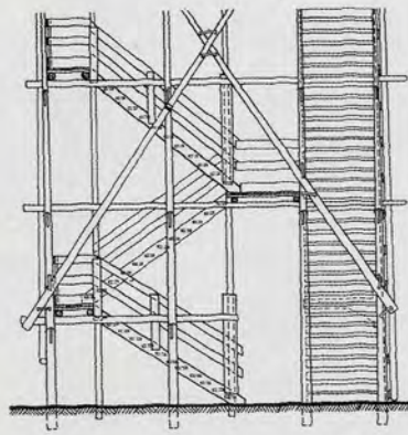
Πρόοψις
