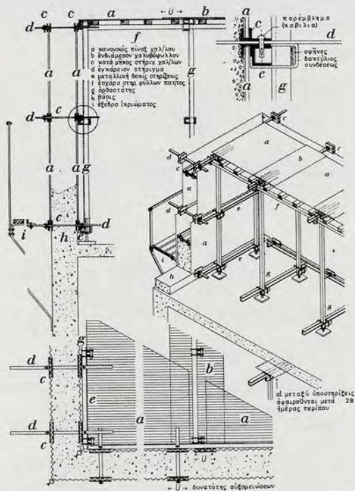
Σχ. 93. Εδούτημα προκατεσκευασμένων μεταλλικών τύπων χυτών τοιχ/ών, εύρεσίτεχνος: LEHMANN.
