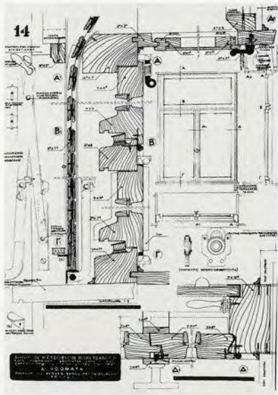
Λεπτομέρεια ξύλινου παραθύρου με ακούρα ρολά
