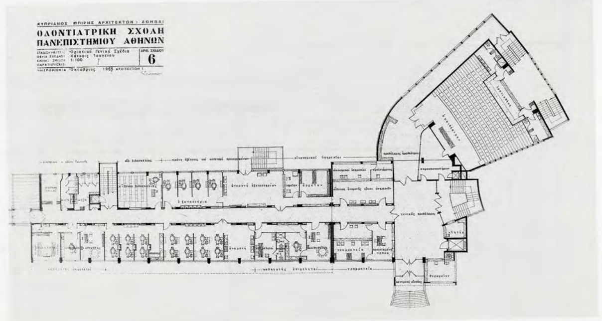
Κάτοψη ισογείου
