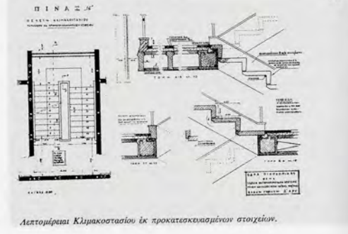
Κλίμακες και Κλιμακοστάσια.
