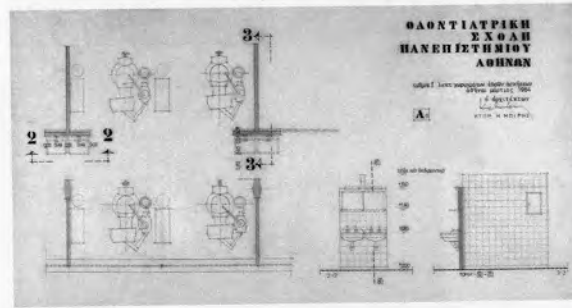
Σχέδιο λεπτομερειών Εργασιών
