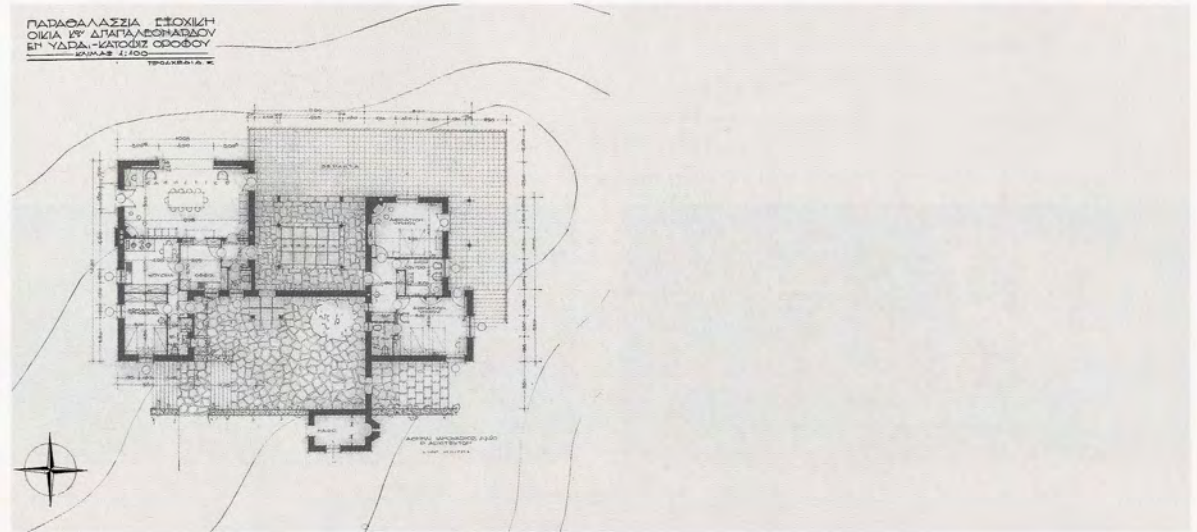
Κάτοψη ισογείου
