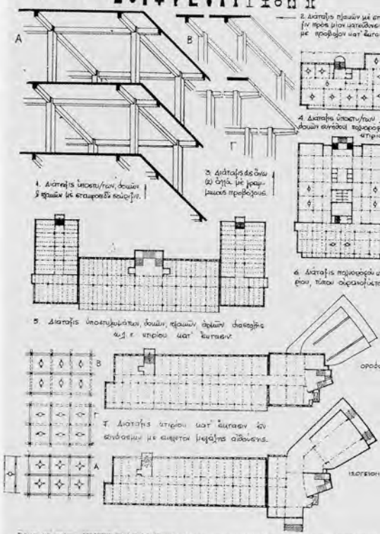
ΠΙΝΑΞ 7. — ΓΕΝΙΚΑΙ ΔΙΑΤΑΞΕΙΣ ΦΕΡΟΝΤΩΝ ΟΡΓΑΝΙΣΜΩΝ ΚΤΙΡΙΩΝ ΥΠΟ ΜΟΡΦΗΝ ΣΤΟΙΧΙΩΝ
