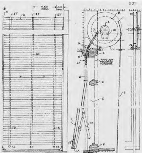
Α. 1:20 Β. 1:10 ΚΑ. 1:10
